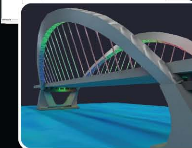
AGI 32
