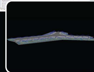
DIALux
